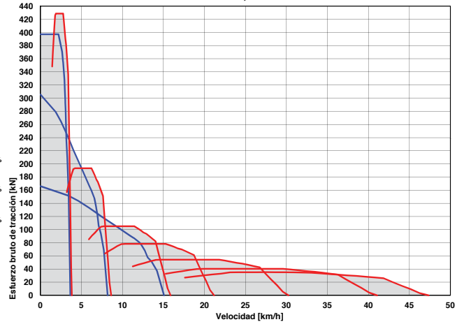
ADT, B60E 4X4 - Esfuerzo de tracción
