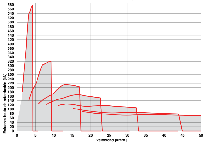
ADT, B60E 4X4 - Retardación
