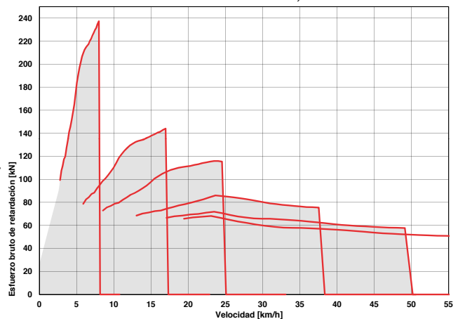
ADT, B35E 6X6 - Retardación
