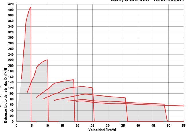
ADT, B45E 6X6 - Retardación
