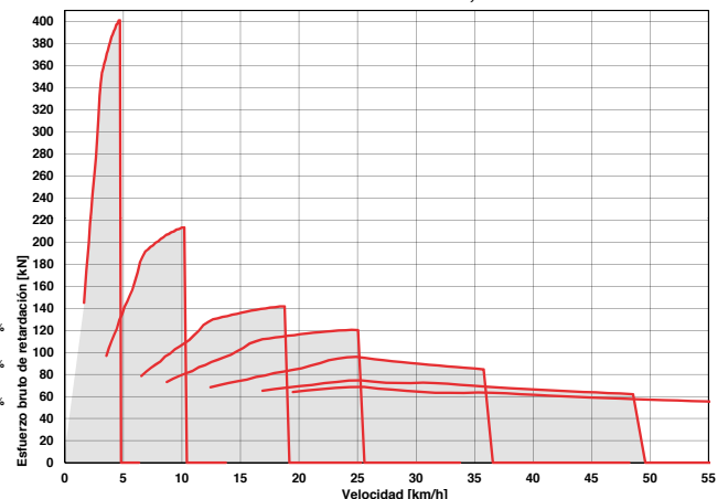
ADT, B40E 6X6 - Retardación
